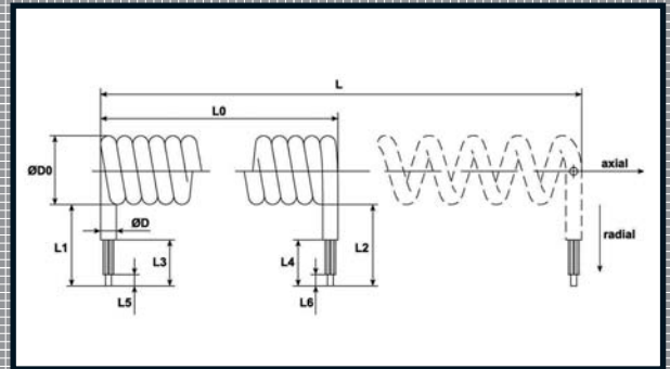
PUR-Mantel Auszugsverhältnis 1 : 6
